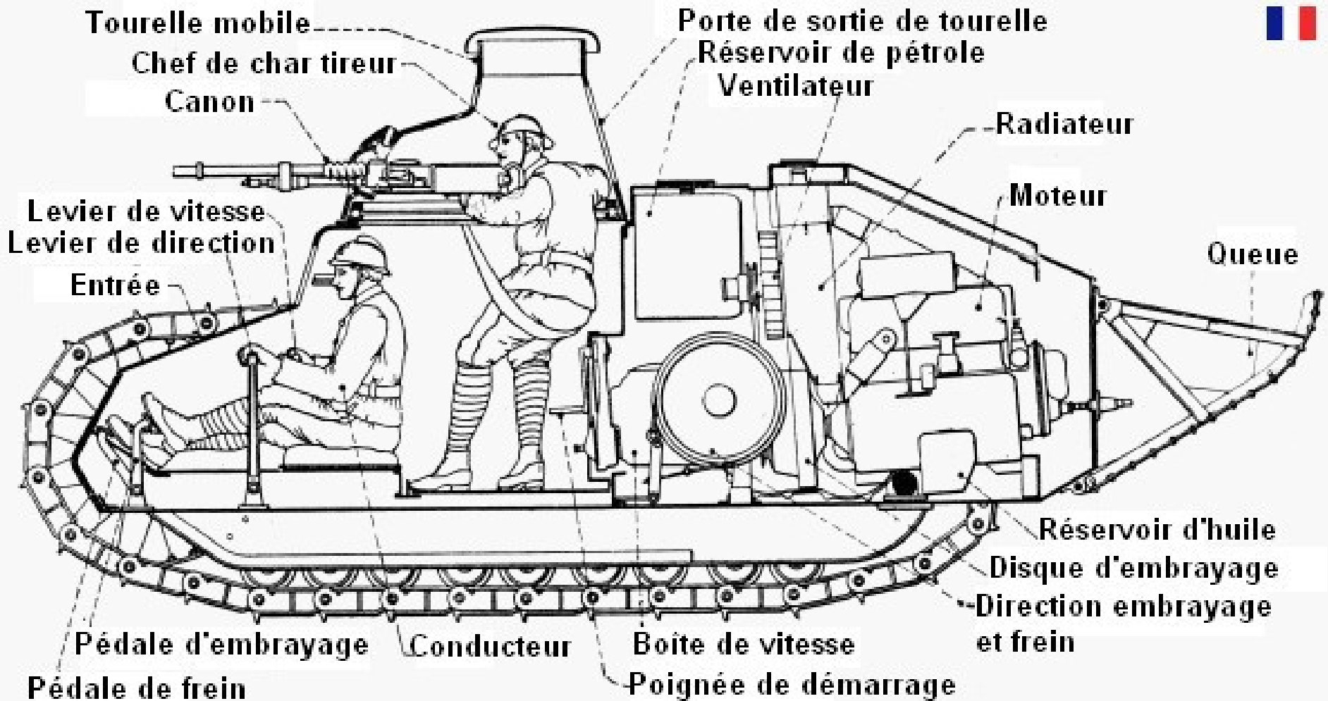
Char Renault FT-17 France diagramme de l'intérieur
